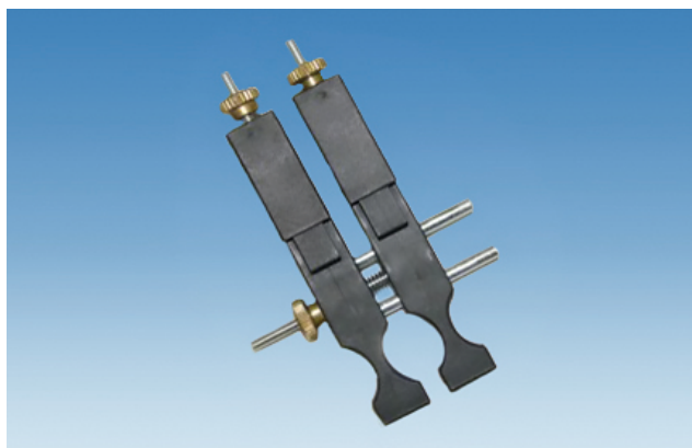
Струбцина для соединения сварных ремней малых сечений
