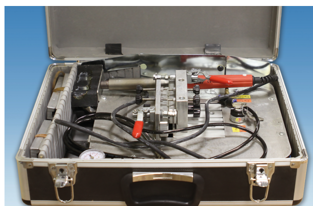
Устройство для соединения сварных ремней внахлест (с перекрытием корда)
