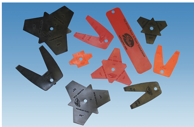
Калибры для измерения сечений клиновых ремней и шкивов
