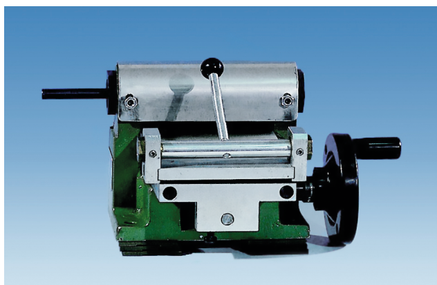
Устройство для шлифовки под клин плоских полиамидных ремней
